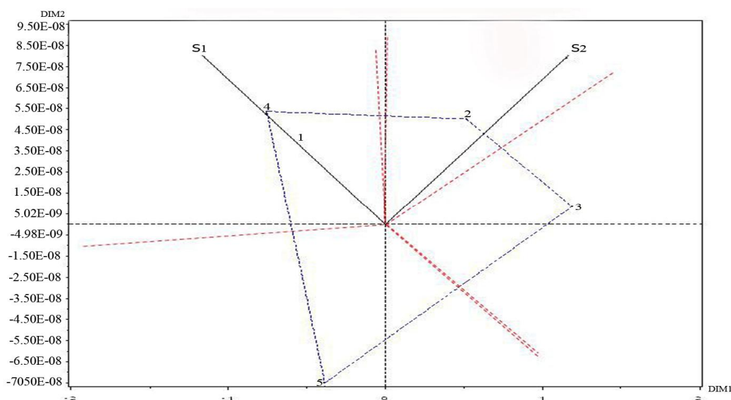
شکل ۳- بای یلات بر اساس مدل AMMI_2 ( S_1 و S_2 به ترتیب دشت و تیر تاش می باشند).
